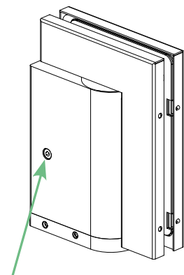
Regelventil für die Türschließgeschwindigkeit.
